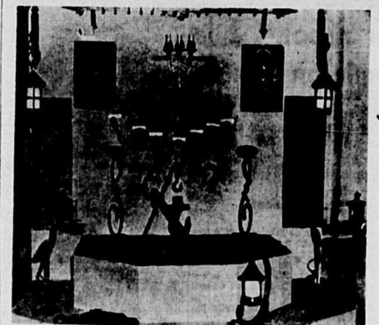
On a pu admirer à l'Ecole technique divers travaux exécutés par les élèves à l'occasion de la fin d'année. On peut voir ci-haut des pièces de fer forgé (lampadaires, candéliers, motifs décoratifs, etc.) (Photo CANADA)
