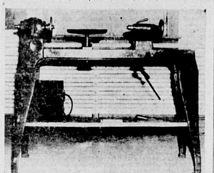
Dans la section d'ajustage, on peut voir un tour à bois, muni d'un moteur électrique fait par les élèves. Ce moteur électrique a une vitesse variant de 1.300 à 3.500 tours à la seconde. (Photo CANADA)
