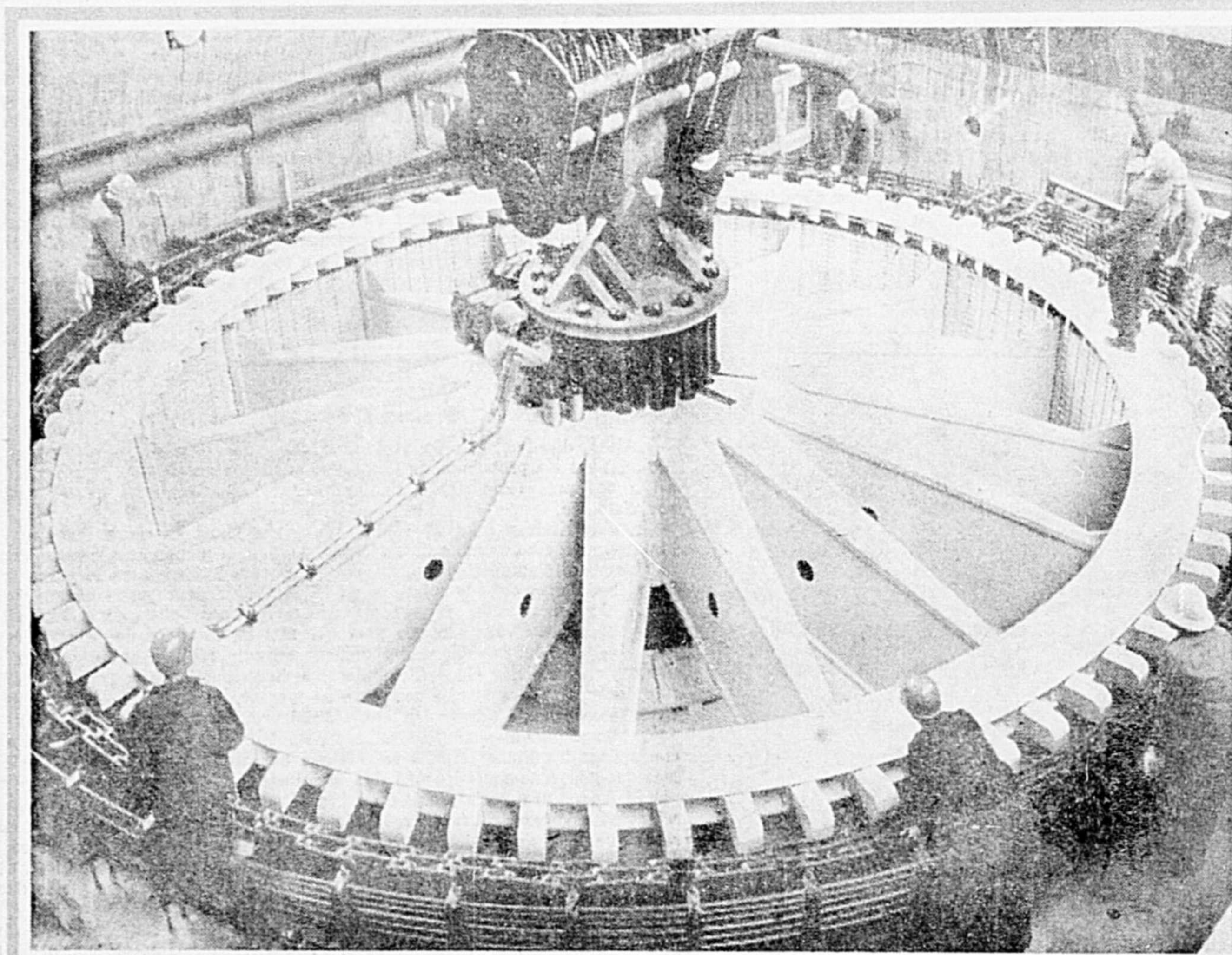
ON INSTALLE LE ROTOR —Le cœur d'un générateur prend place. Ce rotor géant de 225 tonnes tournera bientôt à 106 milles à l'heure pour donner une puis-
