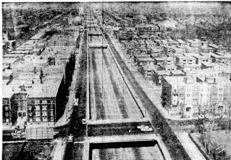
La nouvelle autoroute Décarie, ouverte depuis ce matin, part du Boulevard Métropolitain et va jusqu'au pont Champlain. Pour le moment, deux voies seulement sont ouvertes dans les deux directions. L'autoroute pourra quand même absorber 55,000 véhicules de plus quotidiennement.
