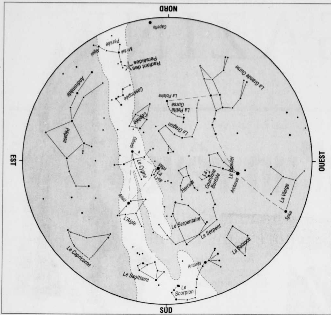
La carte présente le ciel tel qu'on pourra le voir à la mi-août vers 23 h HAE, une heure plus tard au début du mois, une heure plus tôt à la fin. Pour l'utiliser, tenez la carte au-dessus de votre tête, en alignant les points cardinaux. Les lignes pleines identifient les contours des constellations, tandis que le pointillé fin montre les contours de la Voie lactée.
