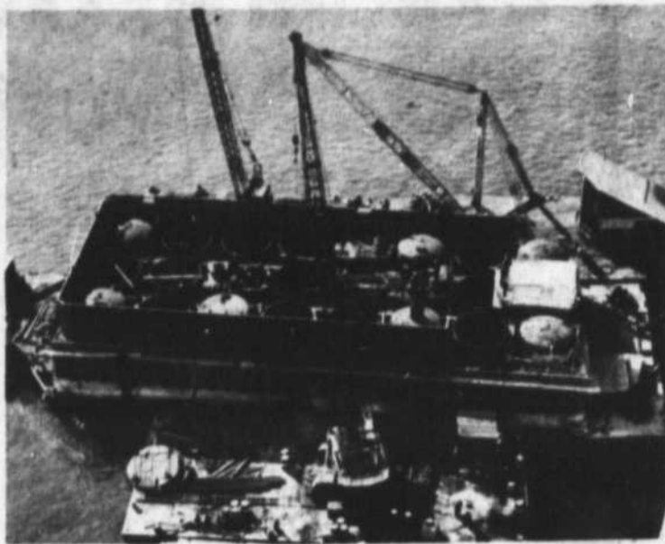
Le pilier S-2 est maintenant une réalité. Du haut de la structure métallique de la rive sud, on voit le coffrage flottant, transporté du quai du Cap de la Madeleine, provenant des chantiers de construction navale de Lauzon. Les ouvriers travaillent actuellement dans les chambres de compression, pour installer les fondations de ce pilier S-2. (Photo Pierre Wibaut)
