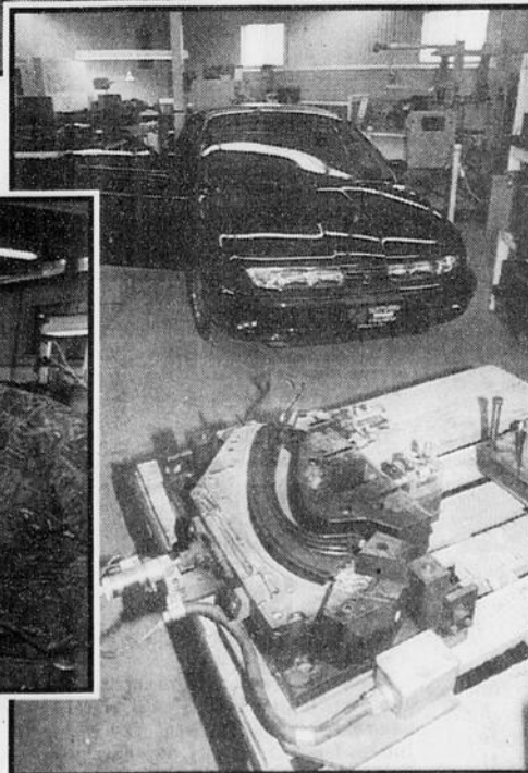
Ici, on aperçoit un moule injection pour les joints d'étanchéité que l'on retrouve sur la Saturn.
