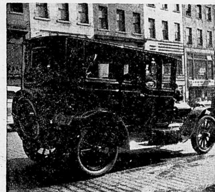
Le Rambler de 1912, modèle Knickerbocker, était une limousine à sept places et entièrement fermée. Un moteur de quatre cylindres lui donnait une puissance de 50 chevaux-vapeur.
