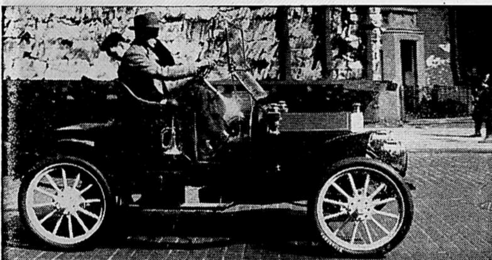
Cette Buick de 1908 fut fabriquée à Flint, dans le Michigan. Il s'agit d'un véhicule doté d'un moteur de 18 chevaux-vapeur. Ses quatre cylindres étaient paillés. Ses phares étaient des lampes à acétylène. Il avait un empattement de 88 pouces.
