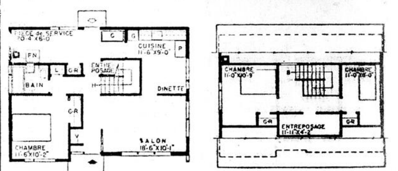
MODÈLES DE PETITES MAISONS LNH — Cette maison attrayante et intéressante d'un étage et demi et sans sous-sol fut dessinée par l'architecte K. R. D. Pratt de St-Vital. Toutes les pièces sont bien éclairées et les fenêtres d'un style particulier ajoutent à l'apparence extérieure agréable.
