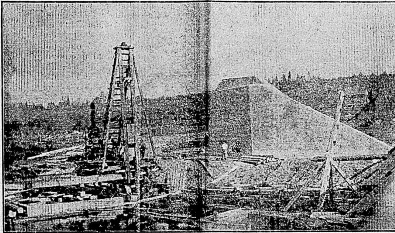
Culée du pont de la rivière Saint-François, vue de profil
