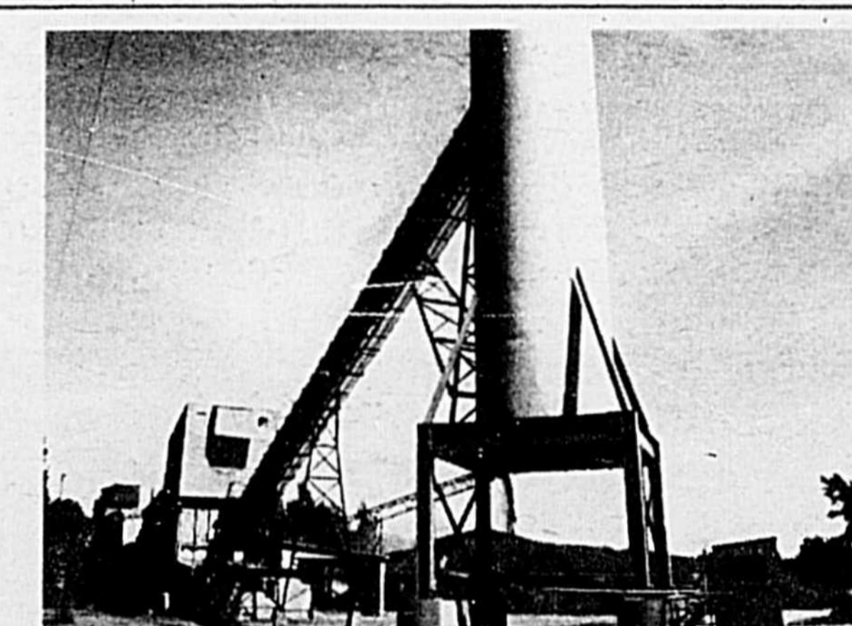
AUJOURD'HUI: Nouveau silo servant à emmagasiner la pierre criblée provenant de l'usine de concassage no. 2.
