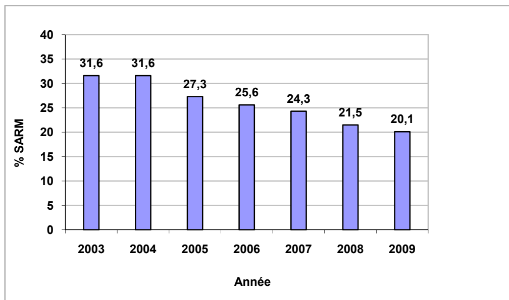
Figure 1 Pourcentage de SARM parmi les bactériémies à S. aureus par année pour tous les centres participants
