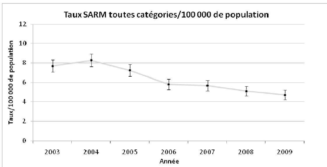
Figure 2 Taux d'incidence de l'ensemble des bactériémies à SARM par 100 000 de population par année de surveillance, 2003-2009
