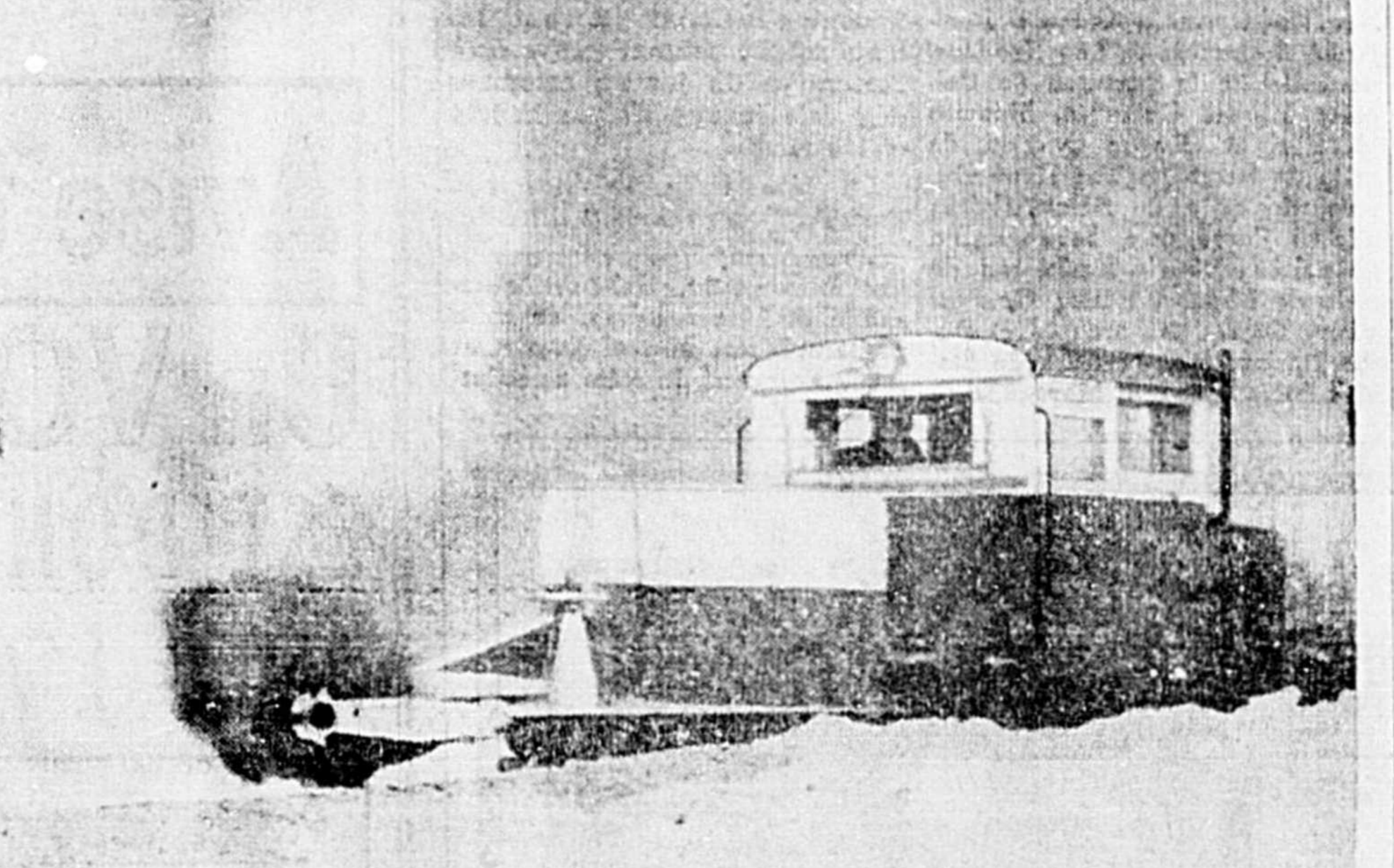
Montées à l'avant d'une locomotive à gazoline de dix tonnes, des brosses rotatives hérisées de rotin balayent tout sur leur passage. Cet équipement mécanisé conserve propres, quel que soit le temps, les neuf milles de voie ferrée étroite qui sillonnent le terrain de l'usine d'explosifs de la C.I.L. à Beloeil.
