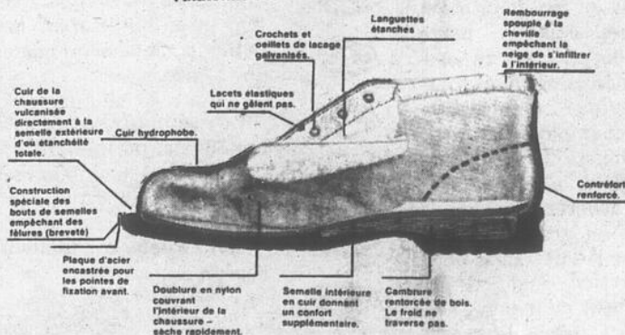
Anatomie des chaussures de ski fonctionnelles Alfa
