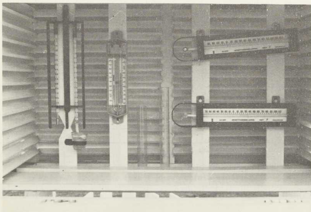
Figure II – Disposition des thermomètres à l'intérieur de l'abri météorologique.
