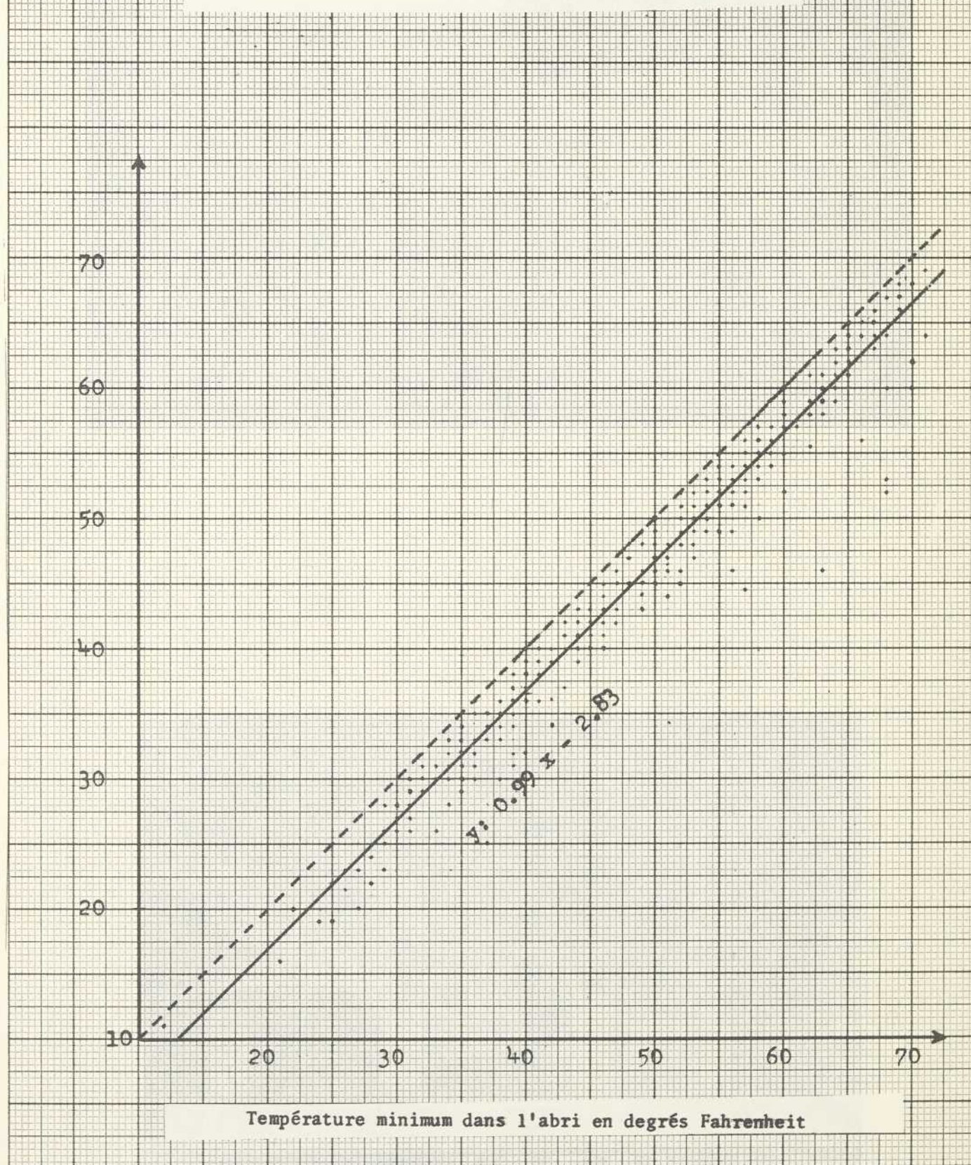
FIGURE III Comparaison des températures minimales dans l'herbe et dans l'abri météorologique à LAPRAIRIE
