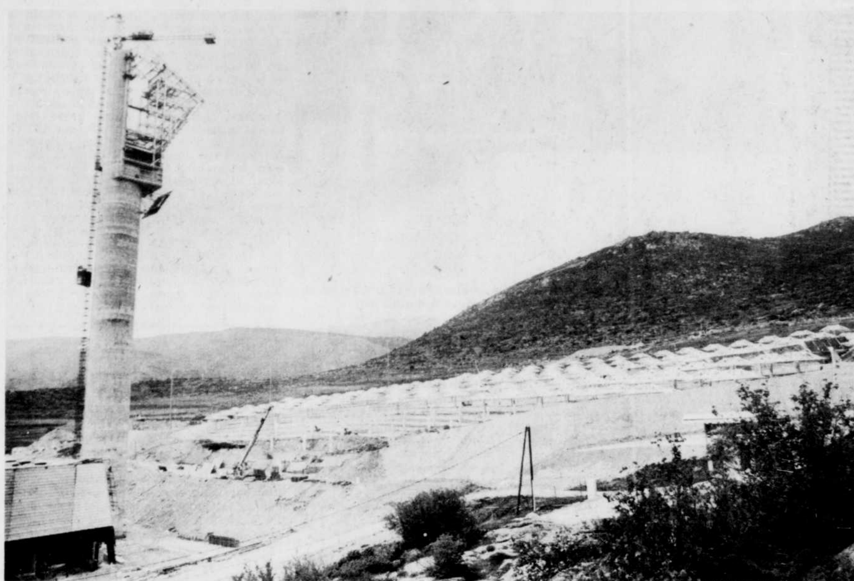
La France s'intéresse également à l'énergie solaire. La première centrale française se trouve à Targassonne dans les Pyrénées orientales.
