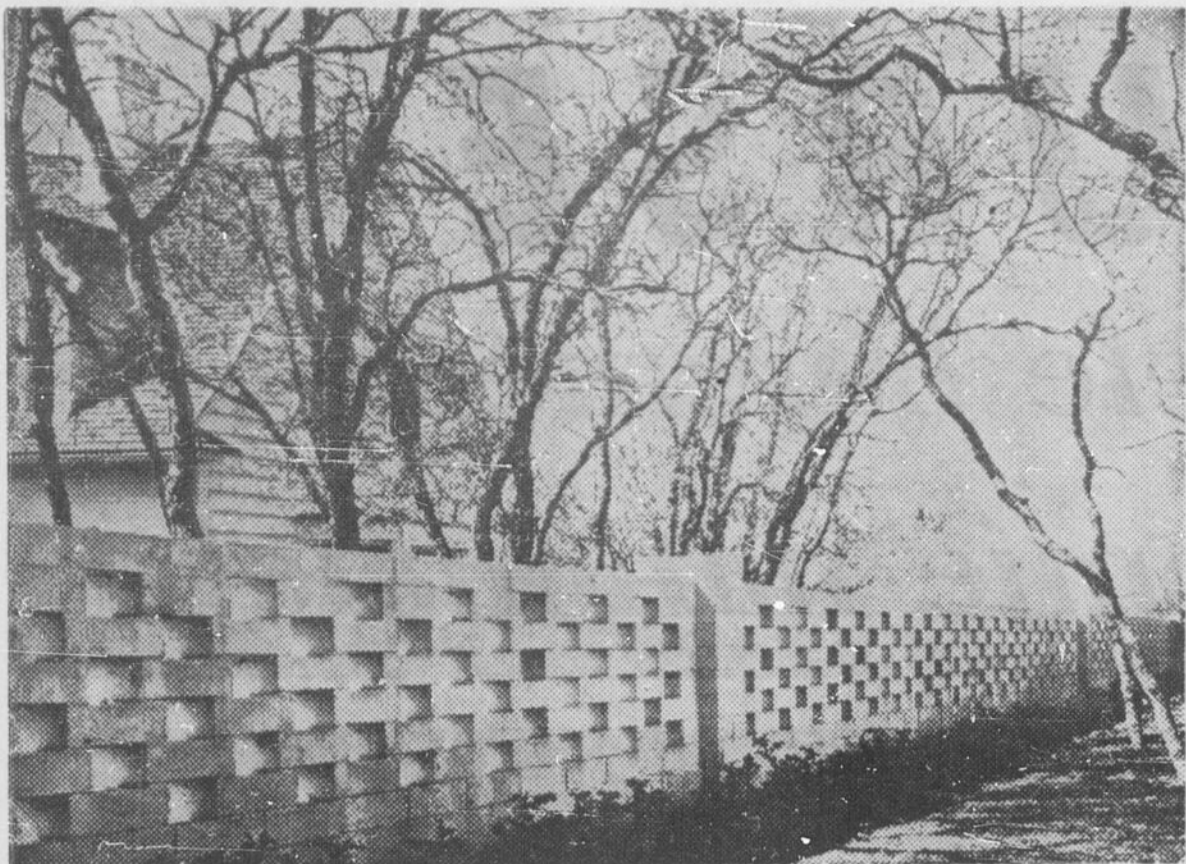
Ce mur genre lattes assure l'intimité tout en laissant passer la brise. Les blocs de ciment se posent vite, ne rouillent ni ne pourrissent, et peuvent résister à la violence des vents et à l'exubérance des enfants les plus agités.
