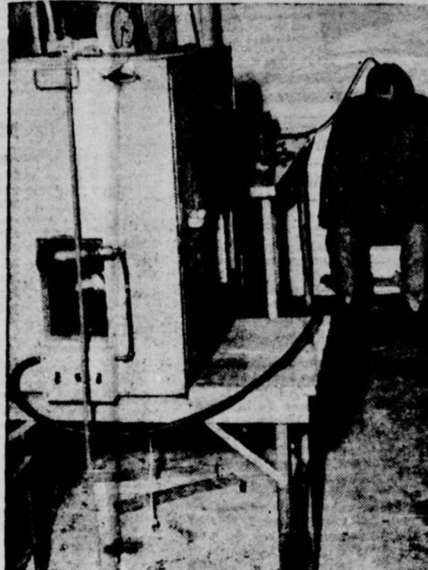
120 OBUS A LA MINUTE.—Bientôt le Canada produira des canons anti-aériens Bofors au complet mais, jusqu'à maintenant nos usines ont fabriqué seulement les tubes amovibles qui s'adaptent à ce genre de canon. Les milliers de tubes ainsi expédiés en Grande-Bretagne ont joué un grand rôle dans la D.C.A. britannique. En effet, le tir rapide des Bofors — jusqu'à 120 obus à la minute — use les tubes rapidement et il faut les remplacer au bout de quelques minutes. A gauche, un ouvrier canadien place un tube dans un tour. A droite, des artilleurs canadiens et leur canon Bofors, "quelque part en Angleterre".
