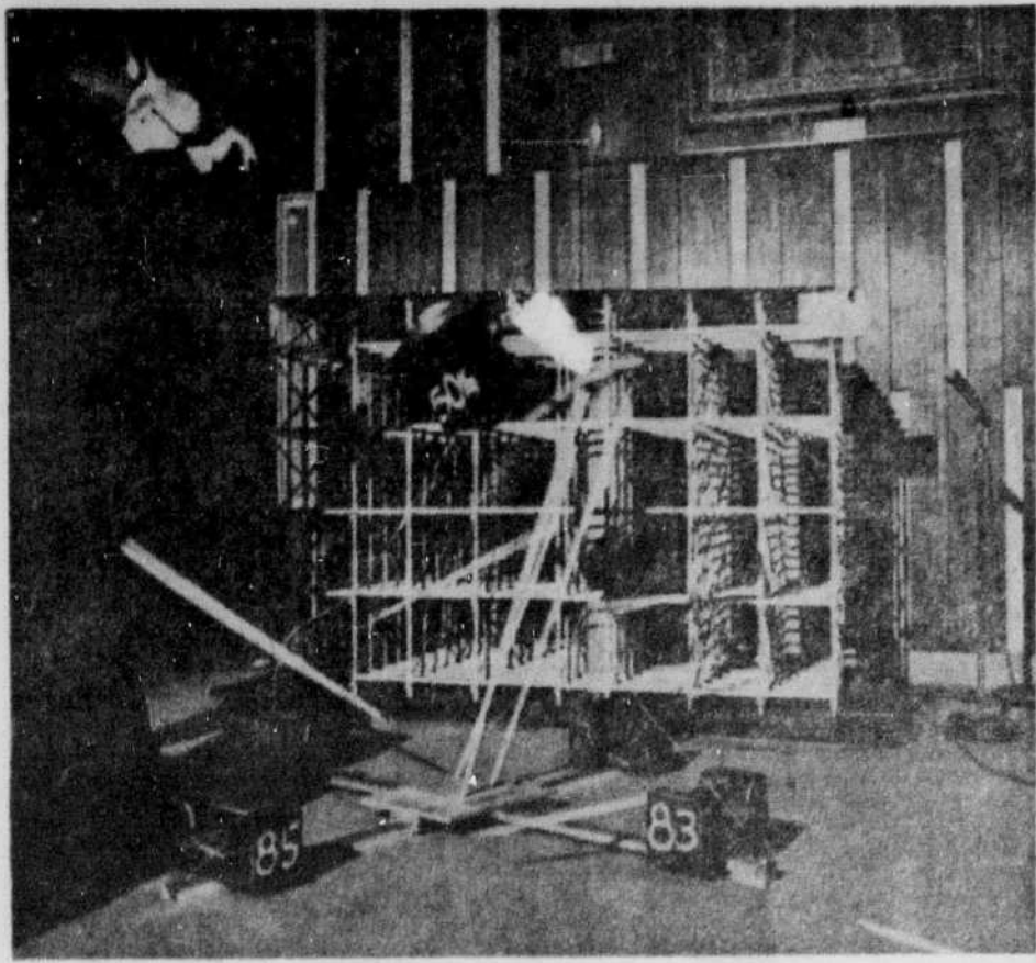
EFFONDREMENT — Le professeur Carson F. Morrison, chef du département de génie civil à l'université de Toronto, a montré lors d'une enquête du coroner hier comment un poids peut casser une charpente si elle n'est pas suffisamment supportée. L'enquête au sujet du pont Heron Road qui
