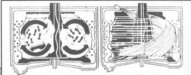
Machine à laver à plusieurs rinçages
