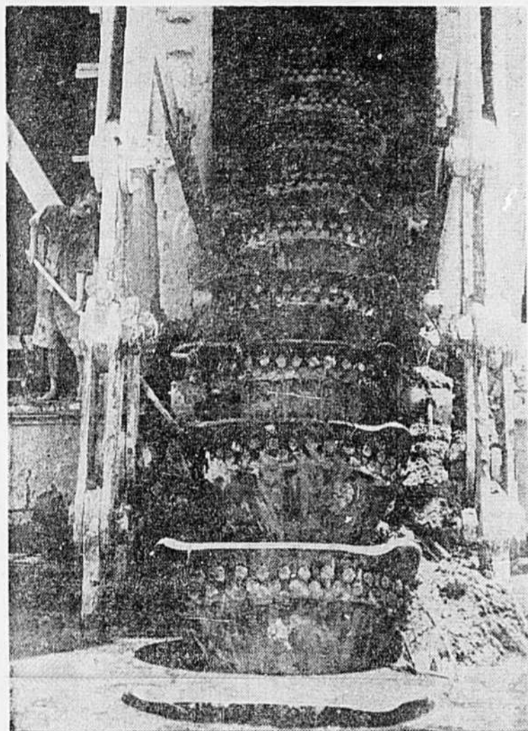
On croit que l'exploitation des mines d'étain en Malaisie remonte à plusieurs siècles. Au 19 e siècle, on découvrit des gisements très riches et les ouvriers chinois affluèrent dans les mines de Parak, de Selangor et de Negri Sembilan. Cette énorme drague dont chaque benne porte 1 tonne et un quart sert à l'extraction du sol contenant le minéral.
