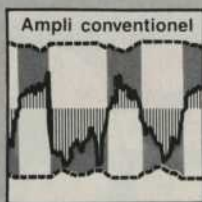
Ampli conventionnel Ligne continue: signal audio. Ligne pointillée: tension de l'alimentation. Zone ombragée: puissance gaspillée. Lignes verticales: puissances aux haut-parleurs.
