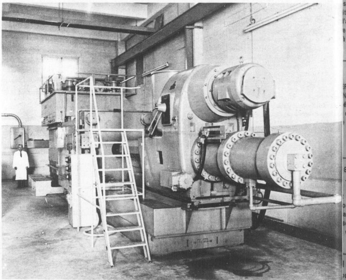
On a, par cette photo, une idée assez juste des dimensions de la nouvelle machine qu'emploient Les Industries Provinciales Ltée pour la fabrication d'objets divers en plastique.
