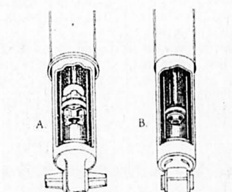
A. Amortisseur arrière de la 505 SR Peugeot et son imposant système de soupapes, qui lui permet de jouer un double rôle - pour le confort, et pour la tenue de route. B. En comparaison, amortisseur arrière de la Cadillac Seville. Chez Peugeot, on insiste aussi sur le fait que chacune des quatre roues est munie d'une suspension indépendante. Ainsi, un dos d'âne au milieu d'un virage, qui ferait faire un écart à une
