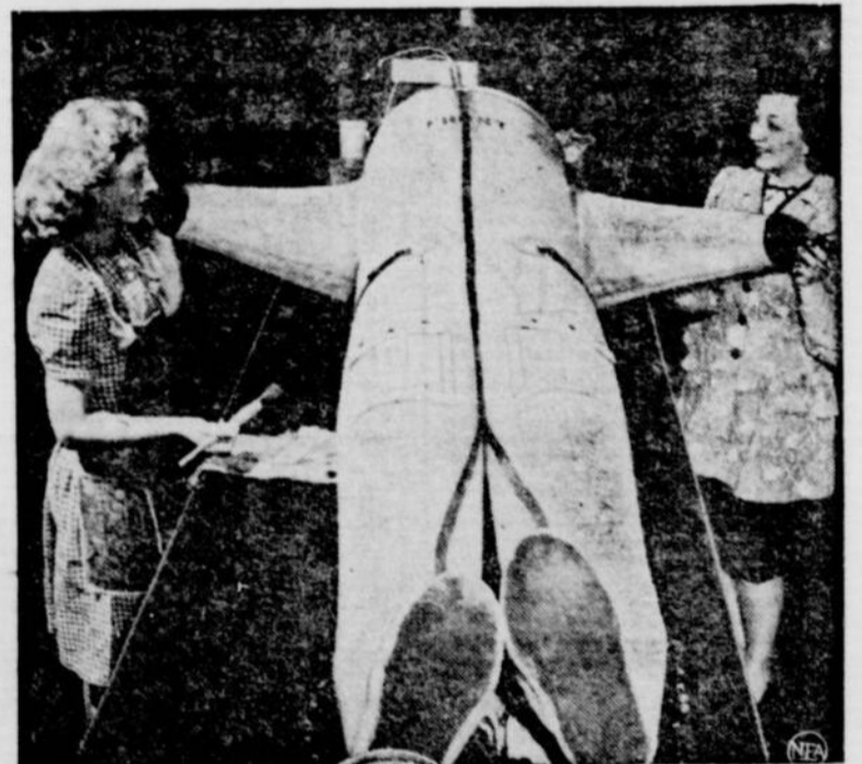
Ce nouvel habit protecteur destiné aux aviateurs obligés d'amerrir dans les eaux glacées ressemble à un monstre marsien. La photographie du haut nous le montre gonflé au cours d'une séance d'inspection. Ci-contre, on le voit tel qu'il apparaît en usage. Imaginé par les ingénieurs de B.-F. Goodrich et les techniciens de la compagnie Wright, cet habit ne pèse que trois livres et s'emploie très facilement.
