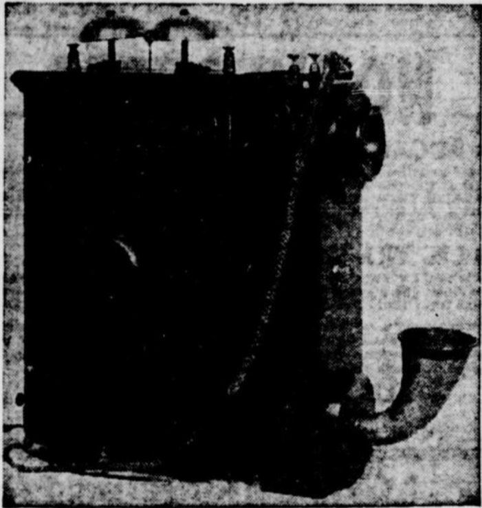
Le téléphone Duquet, considéré comme l'ancêtre de tous les appareils dits micro-combinés ou français, à cause de son emploi répandu en France, fut conçu et fabriqué par Cyrille Duquet, bijoutier de Québec.
