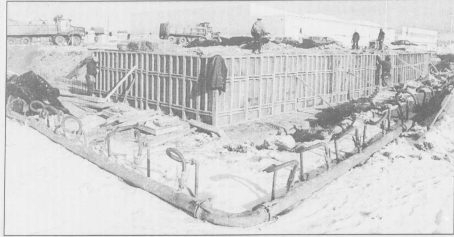
Les travaux de construction du campus de Terrebonne du Cégep régional de Lanaudière ont débuté. On voit ici que le béton a été coulé. Il n'attend plus que les structures d'acier de la future institution. (photo : Gilles Bordonado)
