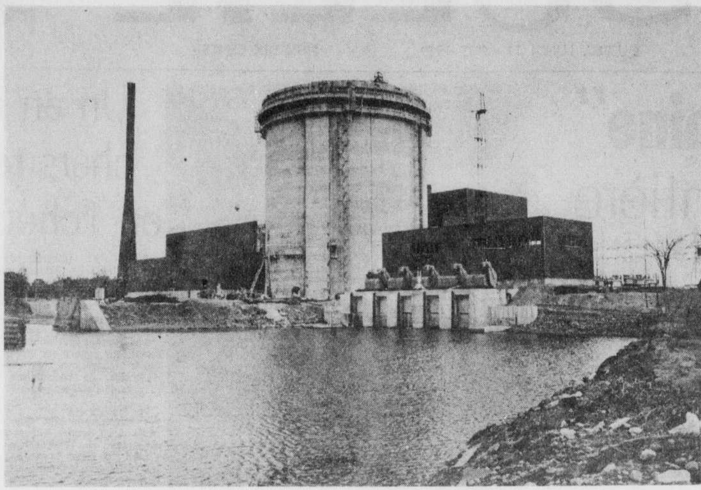
UNE PREMIERE AU QUEBEC — Voici la première centrale nucléaire du Québec, actuellement en chantier sur la rive Sud du St-Laurent, à Gentilly, à une centaine de milles au nord-est de Montréal. La centrale de $106 millions sera
