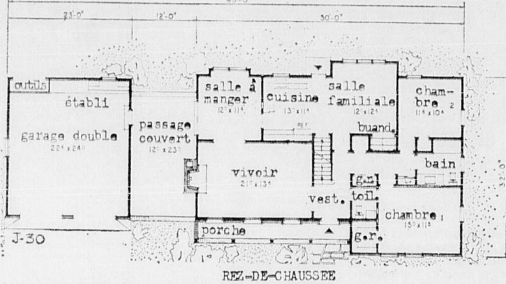
Schéma de la maison J-30
