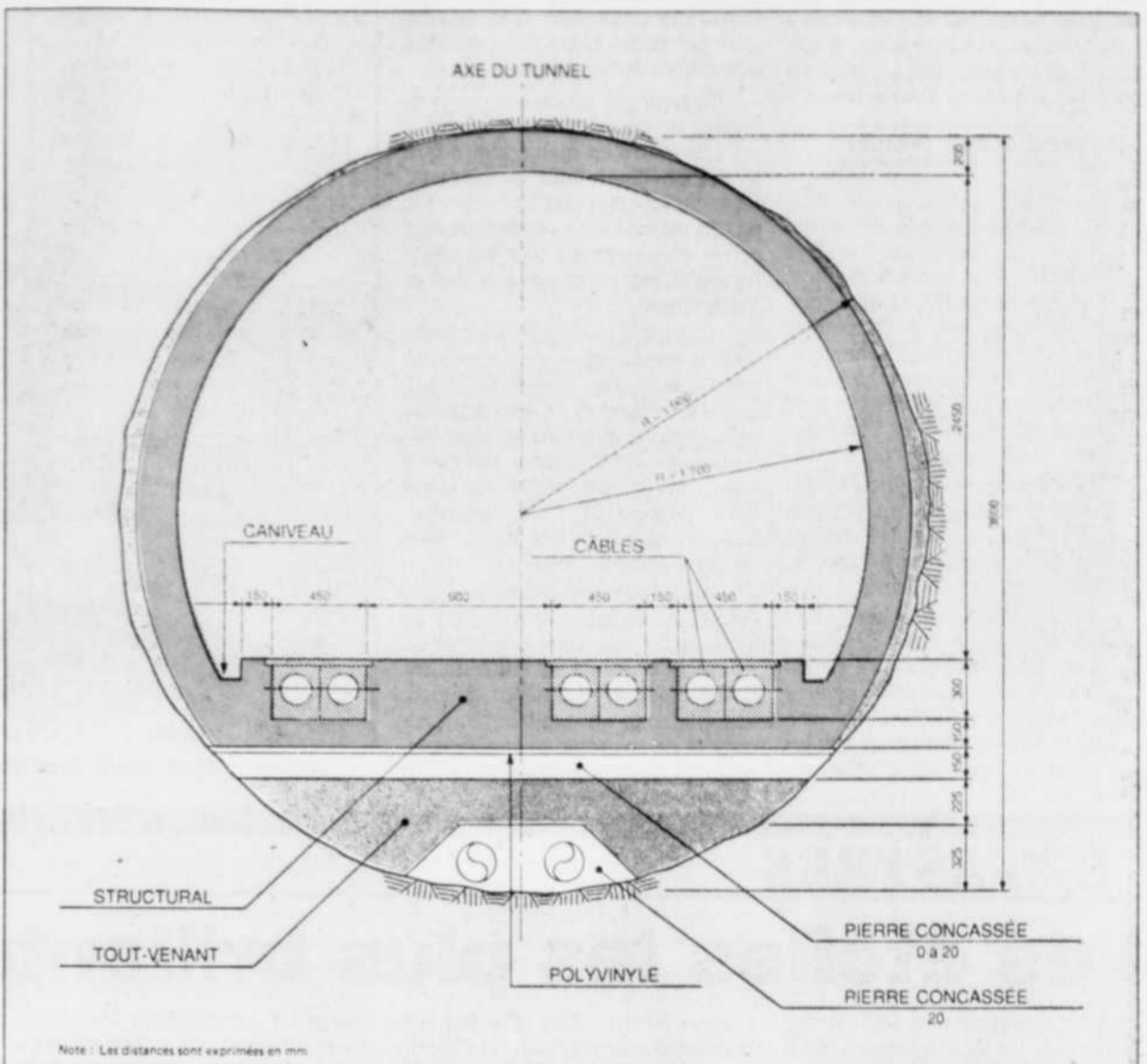
Par le tunnel de quatre mètres de diamètre et long de 4,1 km, six câbles électriques franchiront le Saint-Laurent.
