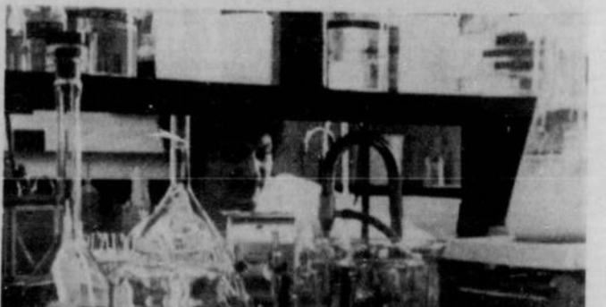
M. Raymond LEPAGE, étudiant gradué, tente de déterminer par analyses chimiques la nature d'un acide nucléique isolé de cellules cancéreuses.
