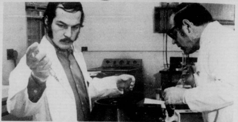
Le Dr. Roger DAOUST, directeur des Laboratoires de Recherche, étudie par des méthodes microscopiques, les changements qui s'opèrent dans les cellules lorsqu'elles se transforment en cellules cancéreuses.
