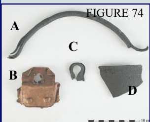
FIGURE 74 Restes de marmites en métal : A) Anse en fer (CgEo-2-4x6-1); B) Oreille d'une marmite en cuivre (CgEo-2-4Z4-2); C) Oreille d'une marmite en fer (CgEo-2-4Z4-3); D) Fragment du rebord d'une marmite en fonte (CgEo-2-5N7-1). (Photographie : Lise Jodoin; infographie : Andrée Héroux)
