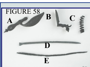
FIGURE 58 Pièces et accessoires de fusil : A) Partie de pontet (CgEo-2-2D6-1); B) Batterie (CgEo-2-10C5-1); C) Tire-bourre (CgEo-2-7F8-1). Tiges de fer à pointe effilée qui auraient pu servir de pointes pour darder les poissons : D) CgEo-2-10F3; E) CgEo-2-10F3; E) CgEo-2-9B2-1. (Photographie : Lise Jodoin; infographie : Andrée Héroux)
