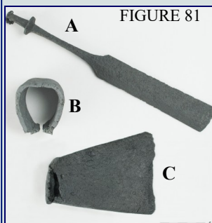
FIGURE 81 Outils servant au travail du bois : A) Ciseau à bois (CgEo-2-4D3-1); B) Tête d'une hache brisée (CgEo-2-4Z3); C) Coin à fendre le bois en fer (CgEo-2-4D3-1). Photographie : Lise Jodoin; infographie : Andrée Héroux
