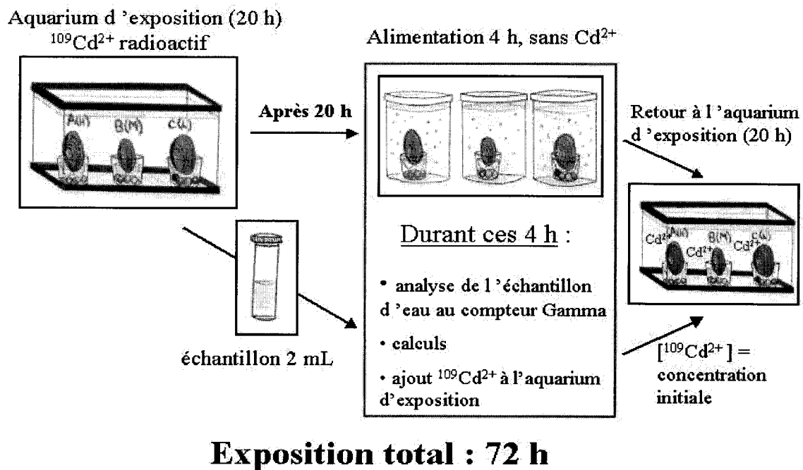
Figure 1. Schéma des étapes d'exposition au Cd 2+ et d'alimentation des bivalves durant les expériences de prise en charge.
