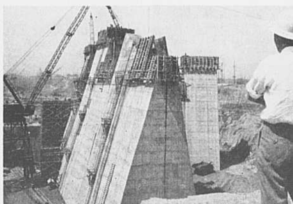
Le contreplaqué de sapin joue un rôle de premier plan en marge du projet de canalisation du St-Laurent, qui reliera l'Atlantique au cœur du pays. Ces gigantesques pyramides de béton armé, parties constitutives de la superstructure d'un centre électrique, ont été moulées avec des formes en contreplaqué de sapin. Lorsque le béton fut déversé dans les formes, les panneaux de contreplaqué soutinrent des pressions allant jusqu'à 700 livres au pouce carré.
