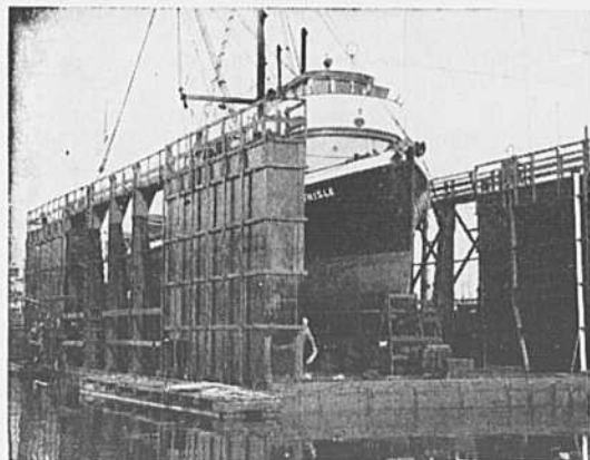
Dans cette cale-sèche de Vancouver, on retrouve les mêmes facultés de rigidité et de résistance à la déformation qui ont permis à l'"Orenda" de surmonter les rafales de l'Atlantique. Les quatre réservoirs de ballast, formant les parois de la cale-sèche, ont été moulés avec des panneaux en contreplaqué de sapin. Après six années de submersions répétées, les réservoirs en contreplaqué n'accusent aucun indice de déformation ou de détérioration.
