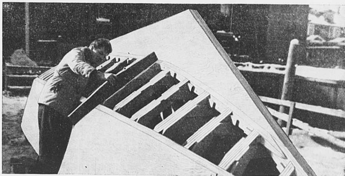
Dans l'arrière-cour de la demeure de Bert Smith, l'"Orenda" prend forme. Smith posa trois panneaux en contreplaqué de sapin à 3 plis, autour d'une charpente, obtenant ainsi une coque de 7/8" d'épaisseur. "En utilisant de vastes panneaux de contreplaqué, mon navire avait moins de coutures et pouvait se garder plus facilement étanche", dit Smith. "J'ai construit huit autres navires avec du contreplaqué et j'ai constaté que la construction en était de beaucoup accélérée".
