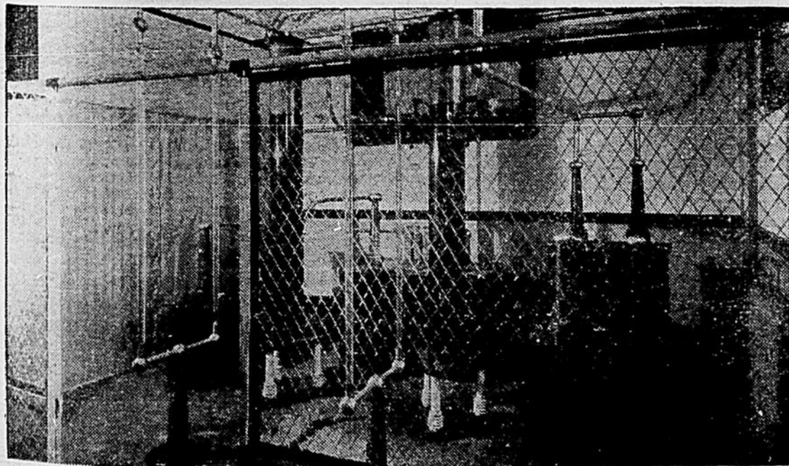
Générateur de l'appareil à 500,000 volts.
