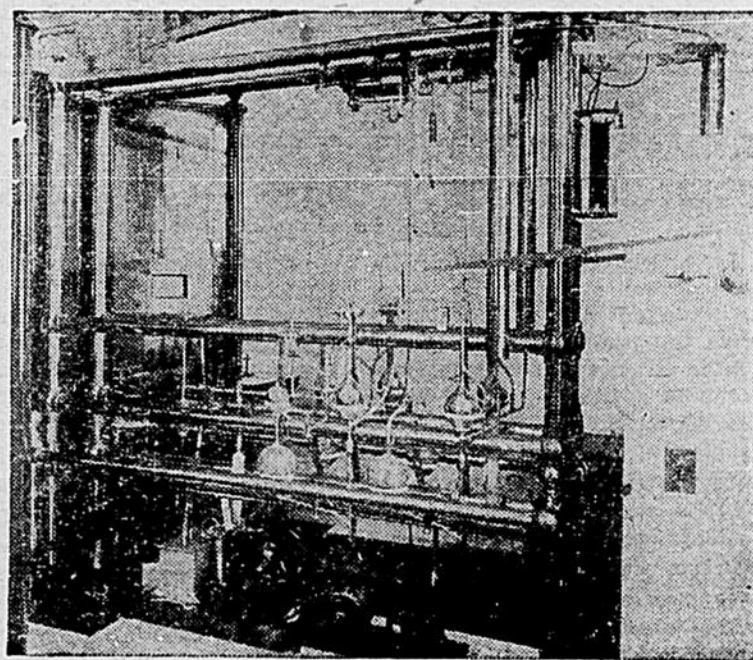
Appareil d'extraction d'émanations du radium.
