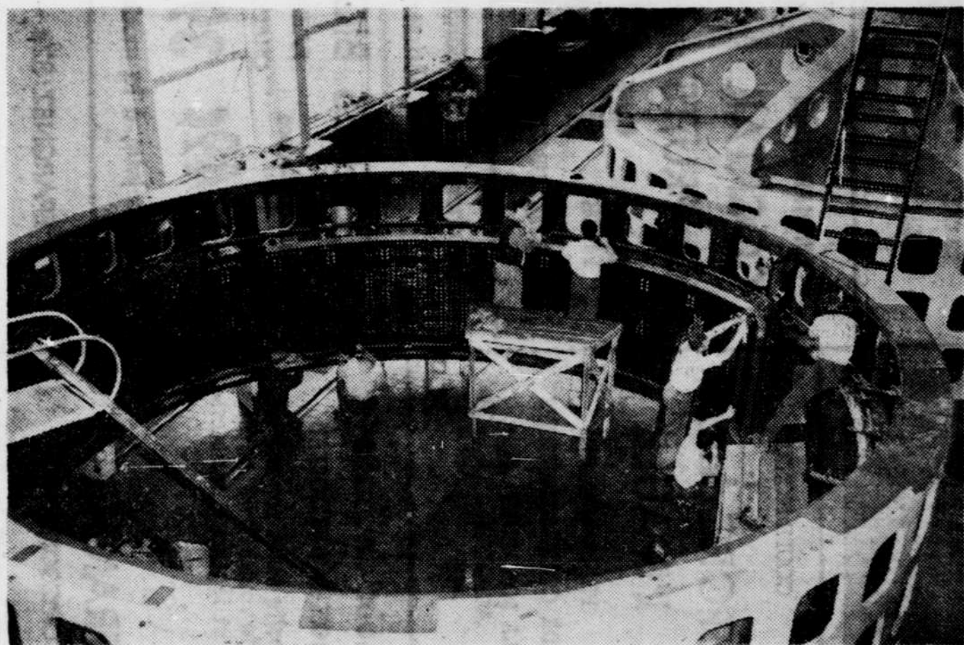
LE STATOR: pièce immense dont le montage demande un temps considérable. Occupés à ce travail, MM. Santori Makila, Onésime Gagnon, Georges Côté,
