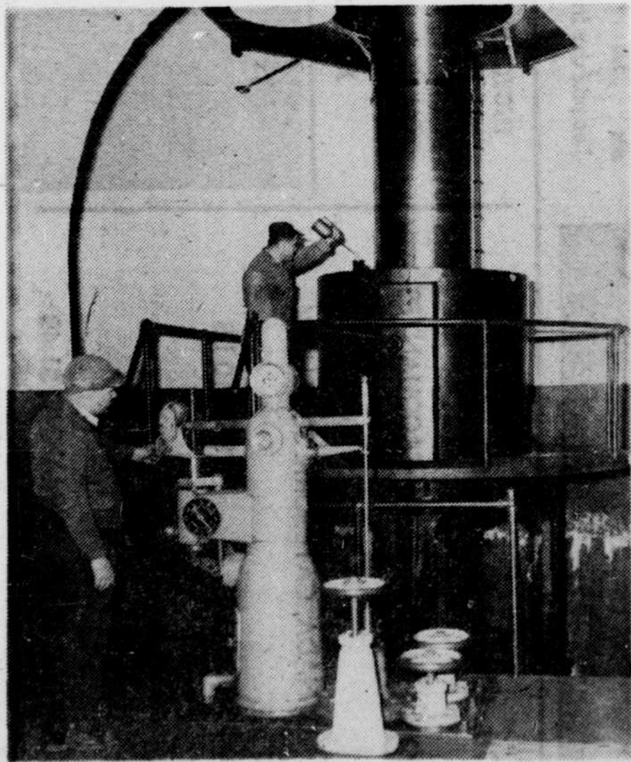
BOULAGE ET AJUSTAGE des pièces de machinerie aussi considérables que celles que l'on trouve dans une centrale hydro-électrique réclament un entretien et une surveillance de tous les instants. Ici, M. Simon Simard huile des engrenages tandis que M. Henri Dionne ajuste le gouverneur.
