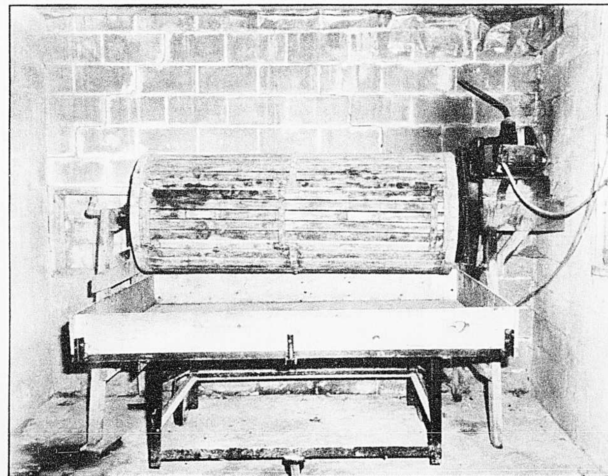
1ère LAVEUSE DE LEGUMES, utilisée dans les années 1930
