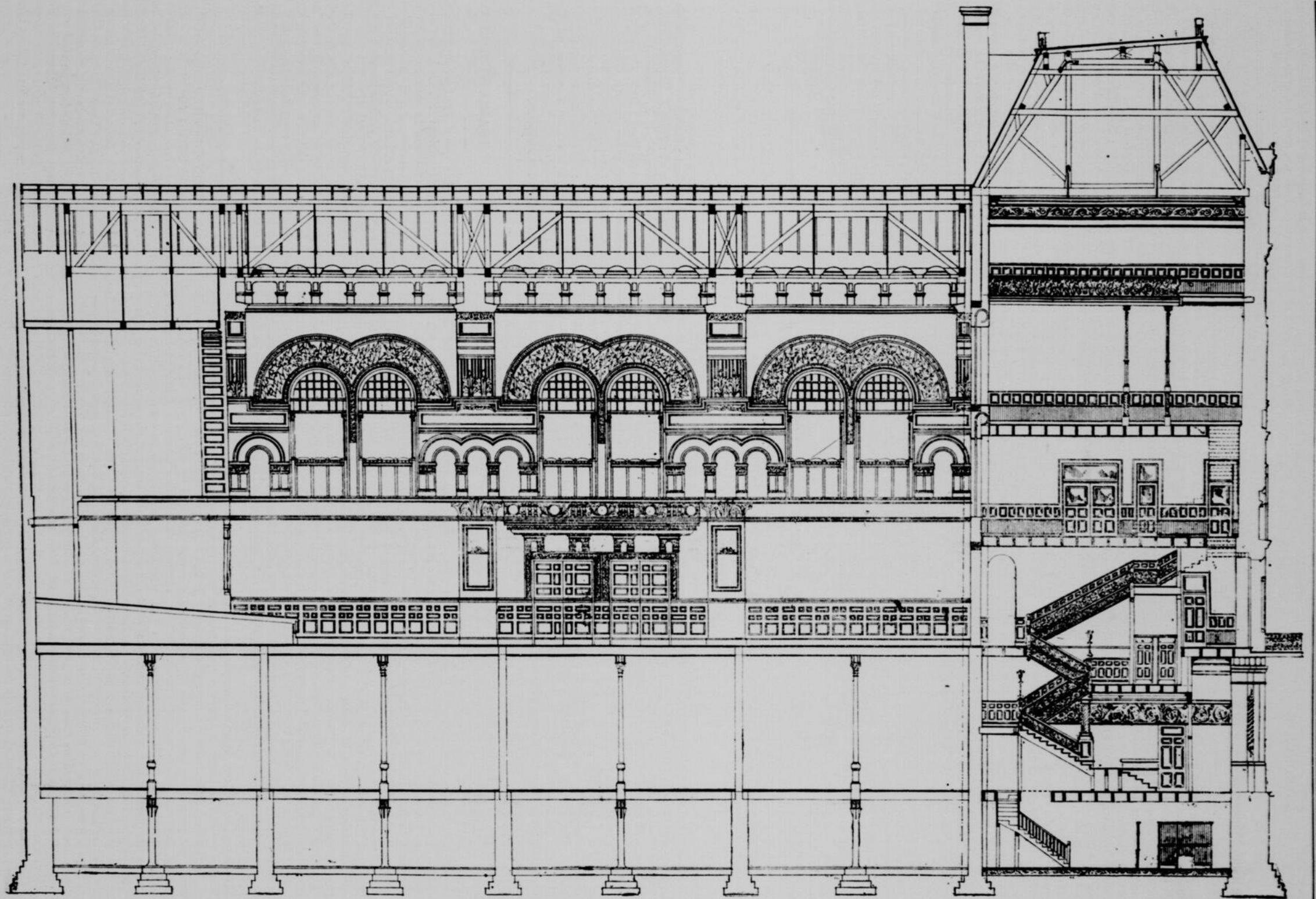
LE MONUMENT NATIONAL. — COUPE LONGITUDINALE
