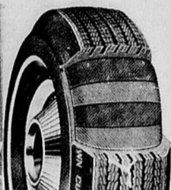
ENTOILAGE EN BIAIS A 4 PLIS DE NYLON
