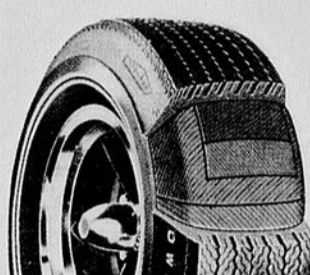
ENTOILAGE EN BIAIS CEINTURE DE POLYESTER FIBRE DE VERRE
