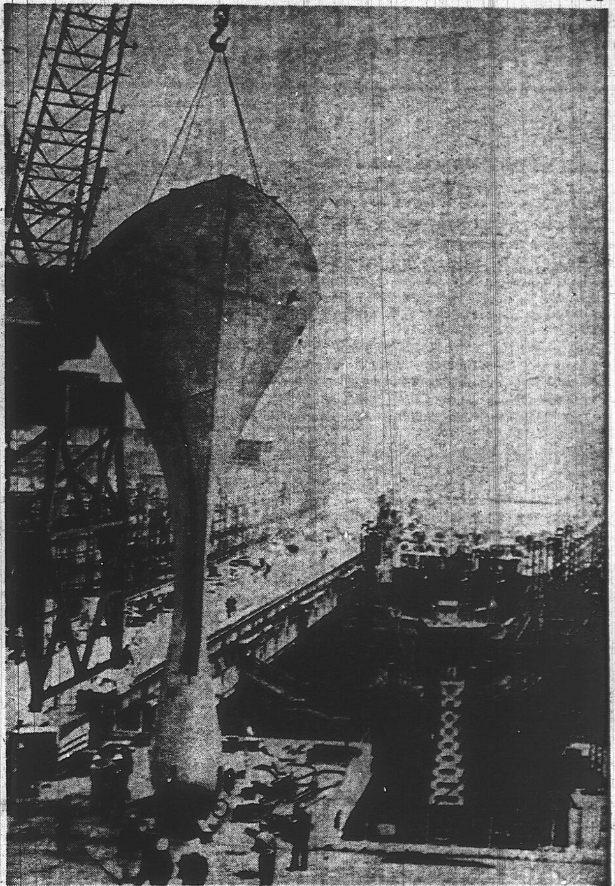
UNE ETRAVE DE 70 TONNES — Une puissante grue soulève et met en place l'étrave géante du navire de guerre atomique "Long Beach" en chantier à Quincy. Ce sera le premier navire de surface propulsé par la force atomique. Il mesure 721 pieds de long. Il sera lancé et baptisé le 20 juin. (Fac-similé UPI — "Montréal-Matin")
