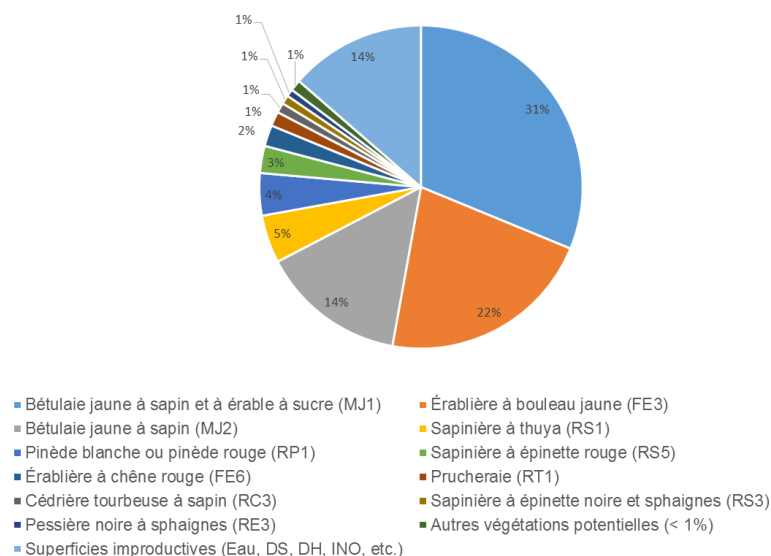
Figure 2 - Principaux types de végétation potentielle trouvés dans l'UA 081-51
