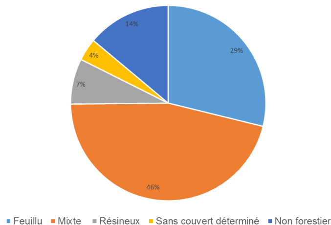
Figure 3 - Importance des différents couverts forestiers de l'UA 081-51
