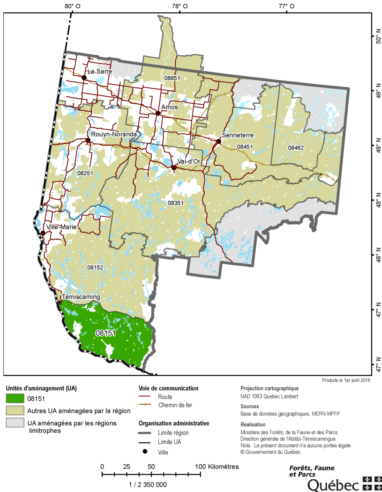
Carte 2 - Localisation du territoire de l'UA 081-51 au PAFIT 2018-2023
