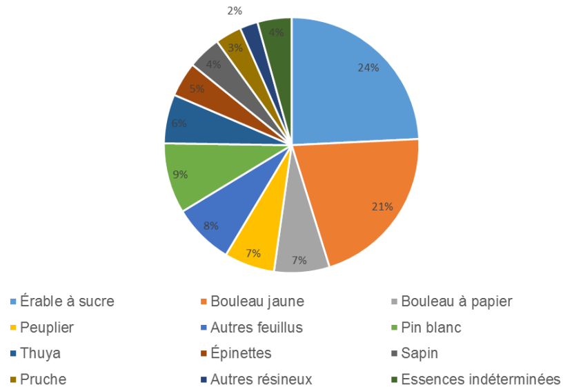
Figure 4 - Importance des différentes essences de l'UA 081-51 29
