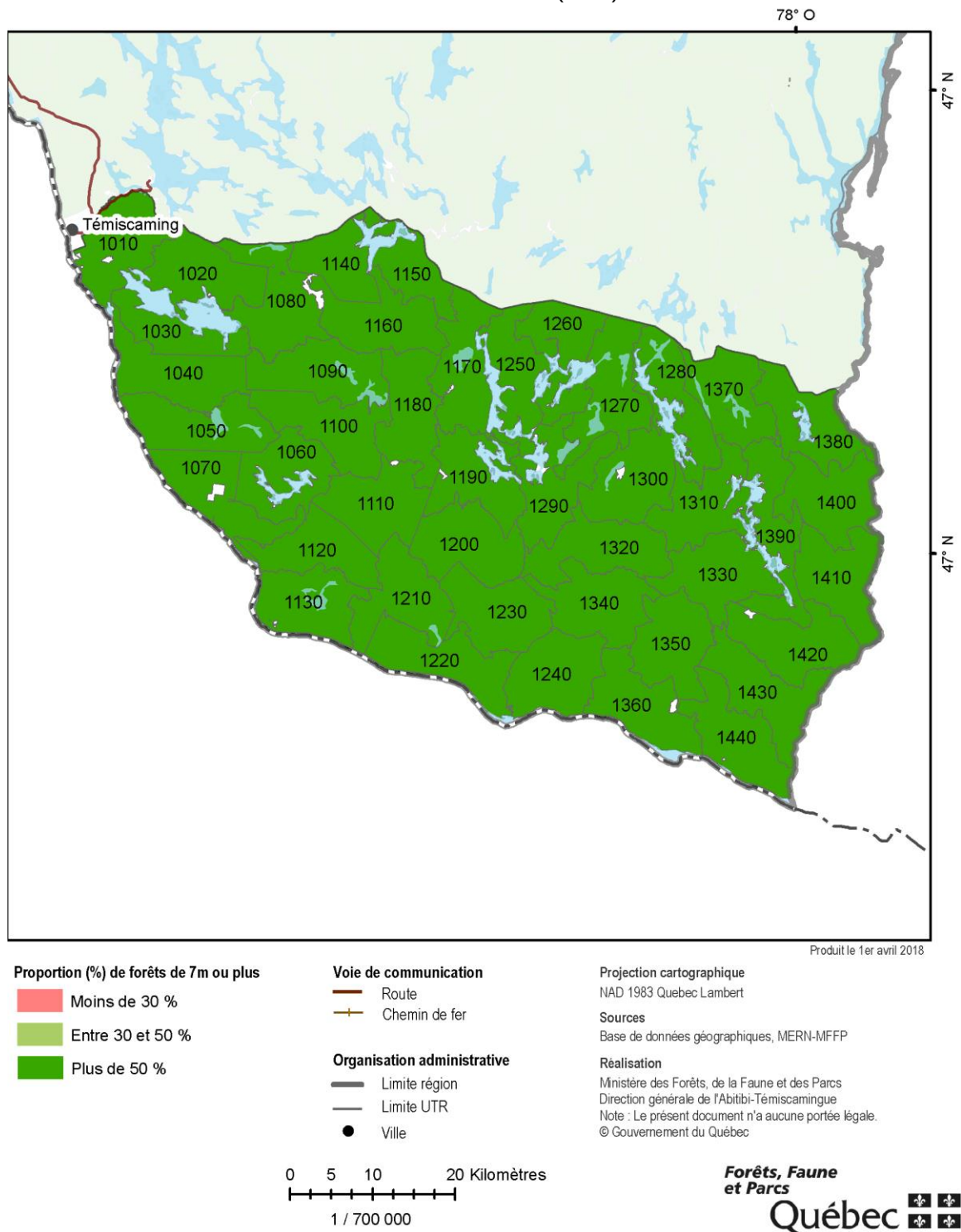
Carte 3 - Portrait des unités territoriales de référence (UTR)
