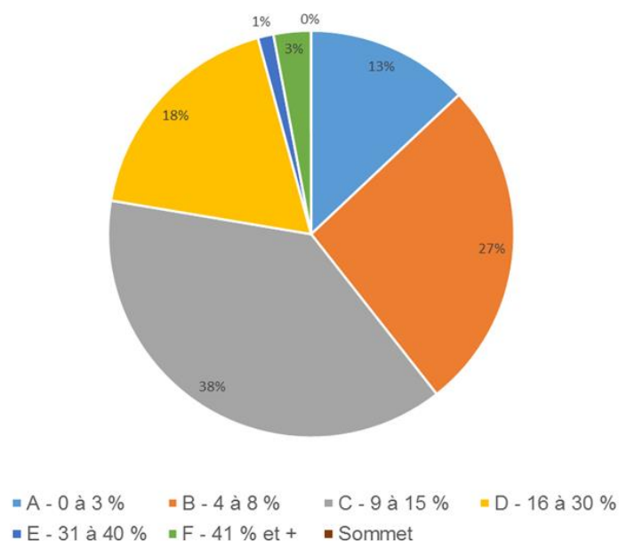
Figure 6 - Classes de pente de l'UA 081-51 au PAFIT 2018-2023
