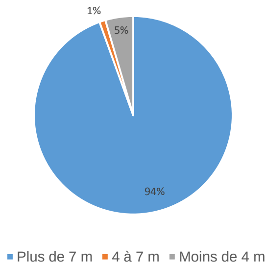
Figure 5 – Stades de développement des peuplements
