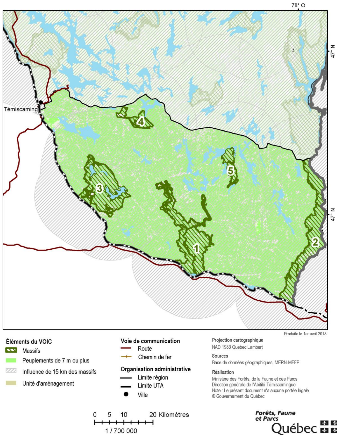
Carte 12 - Massifs forestiers sélectionnés pour la période 2018-2023
