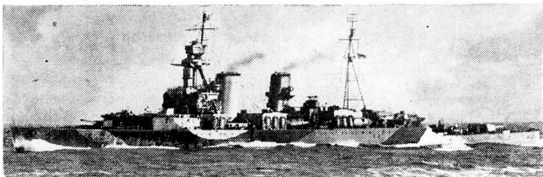
Le "Frobisher", un croiseur britannique de la classe "Hawkins". Armement: sept canons de 7.5 pouces, quatre canons antiavions de 4 pouces, quatorze canons de petit calibre et quatre tubes lance-torpilles de 21 pouces. Déplacement: 9.860 tonnes. Effectif au complet: 712 à 729 officiers et marins. Dimensions: longueur, 665 pieds; largeur maximum, 65 pieds.
