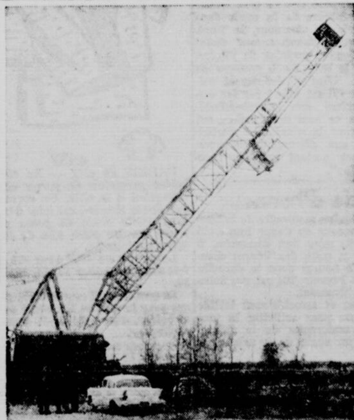
Un puissant derrick rotatif apporte maintenant son concours à la recherche du pétrole dans les basses-terres du St-Laurent. On voit ici cet imposant outillage avant et pendant qu'on dresse la tour haute de plus de 100 pieds. Il est à l'oeuvre depuis quelques jours sur la rive même du fleuve, face aux Trois-Rivières, sur la terre de M. Armand Gauthier, de St-Grégoire. Il foncera des puits que des derricks à percussion avaient commencé de forer. La compagnie Lowlands Exploration, filiale de l'Imperial Oil, exécute ces travaux.
