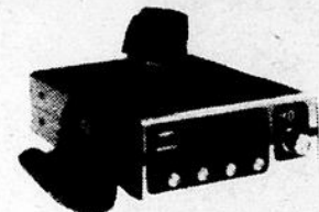
MPL5-77 EMETTEUR - RECEPTEUR CITIZENS AM/SSB 40 CANAUX
