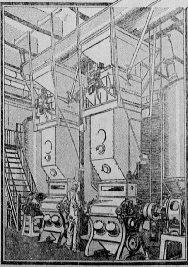
Les concasseurs à malt de la Brasserie Dow, Montréal
