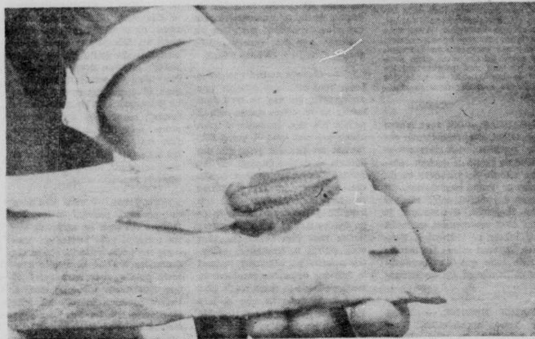
La trouvaille. Un coup de pic a fait éclater une pierre sédimentaire qui renfermait un beau fossile. Le spécimen a été trouvé à Courville par le jeune André Larue. Il s'agit d'un trilobite, genre de crustacés qui vivaient dans les mers à l'âge géologique primaire, il y a des centaines de millions d'années. (Photo Rolland Dumais)
