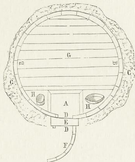
Plan à terre d'une Iglo- çiyoaçk ou hutte de neige servant de campement en voyage.
