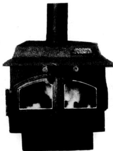
Poêle à bois VAGABOND de SELKIRK
