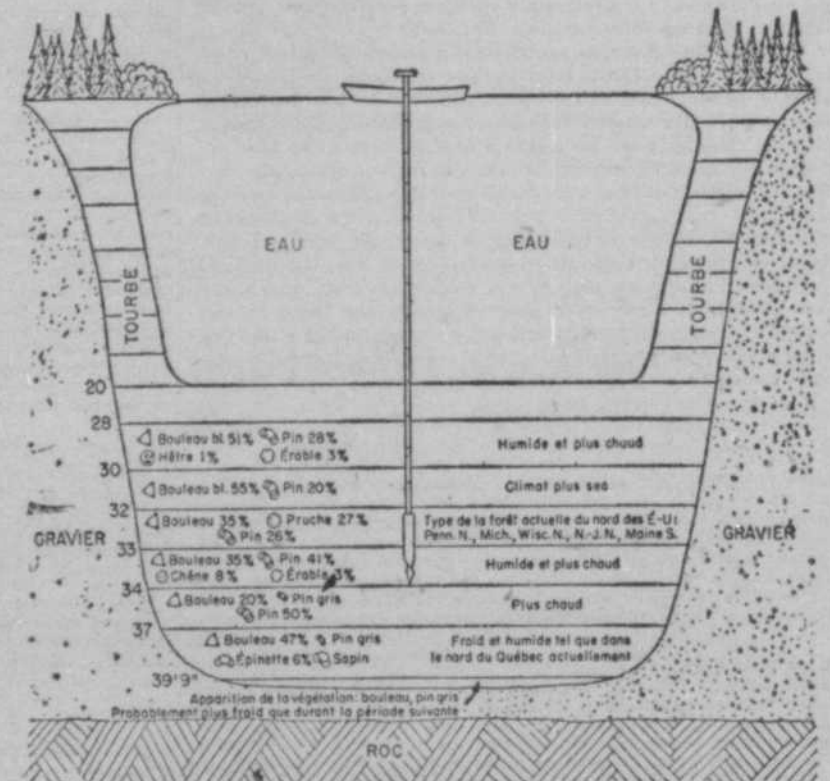
Coupe schématique du lac aux Atocas, montrant la succession des associations forestières et les variations du climat depuis la glaciation.
