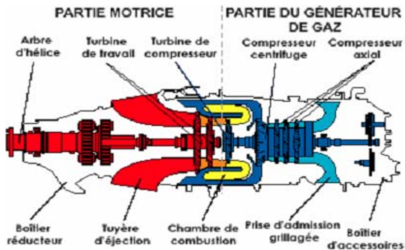
Figure 4.5: Structure du moteur PT6A (gracieuseté de P&WC)
