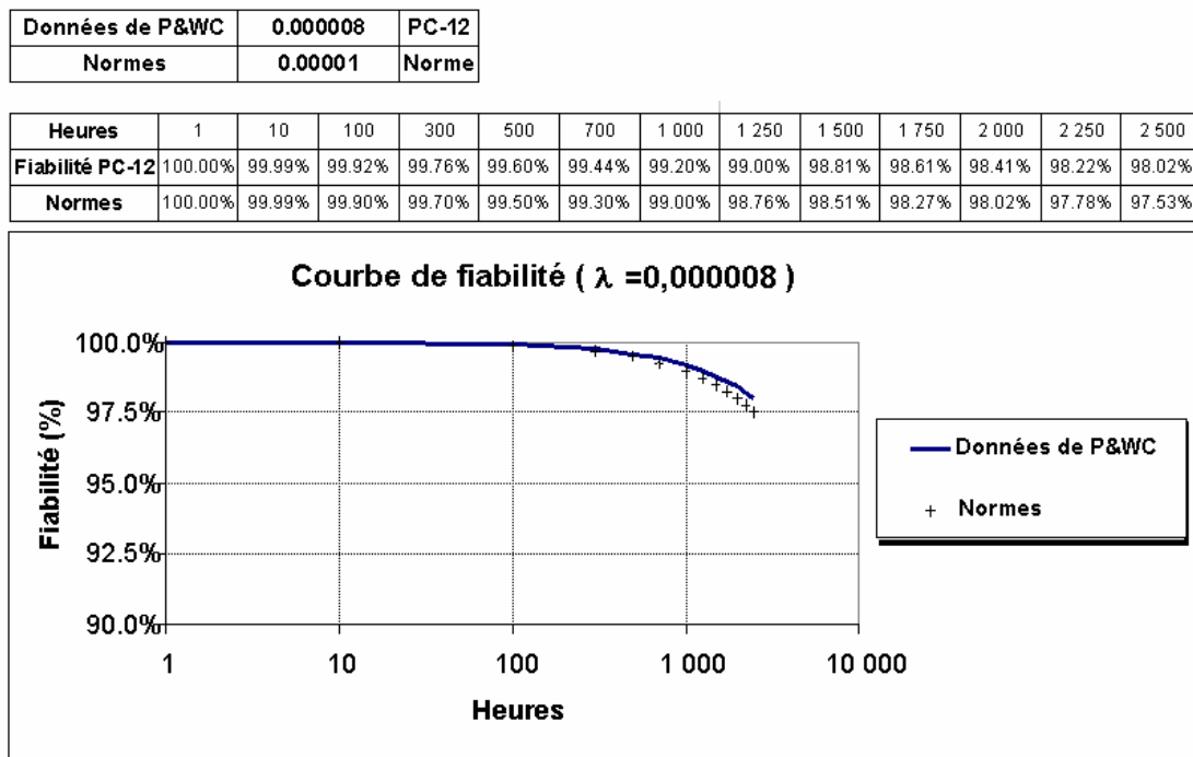
Figure 7.1 Courbe de fiabilité du moteur du PC-12 ( \lambda=0,000008 )
