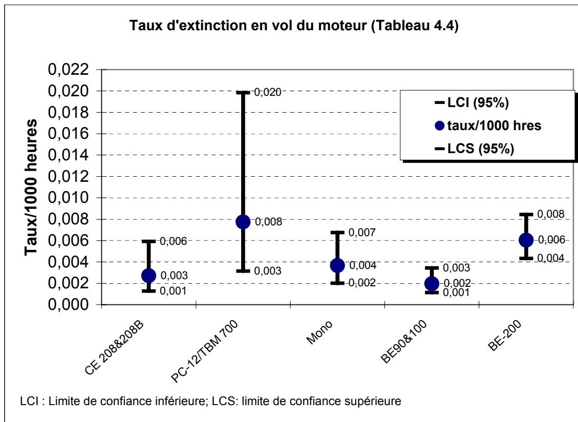
Figure 4.5: Taux d'extinction en vol des moteurs PT6A (2000-2002)
