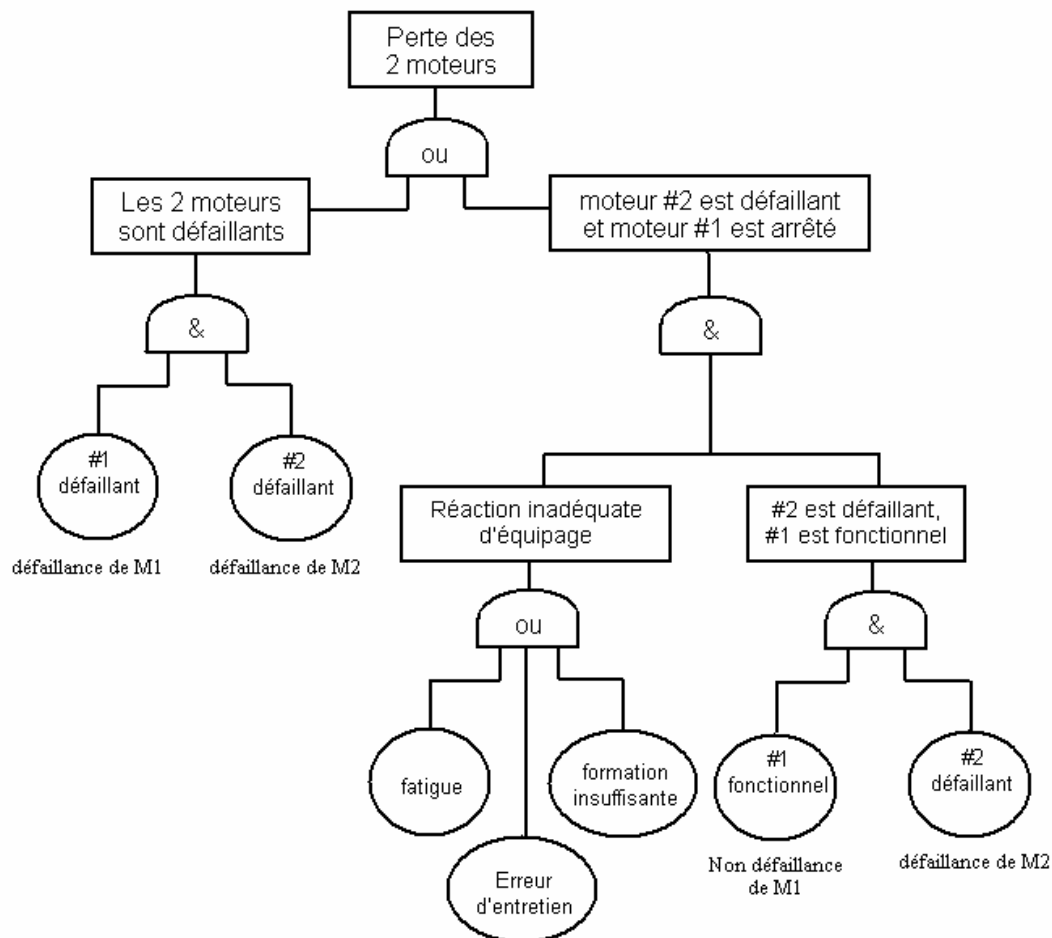
Figure 4.1: Modes de défaillances pour le bimoteur.
