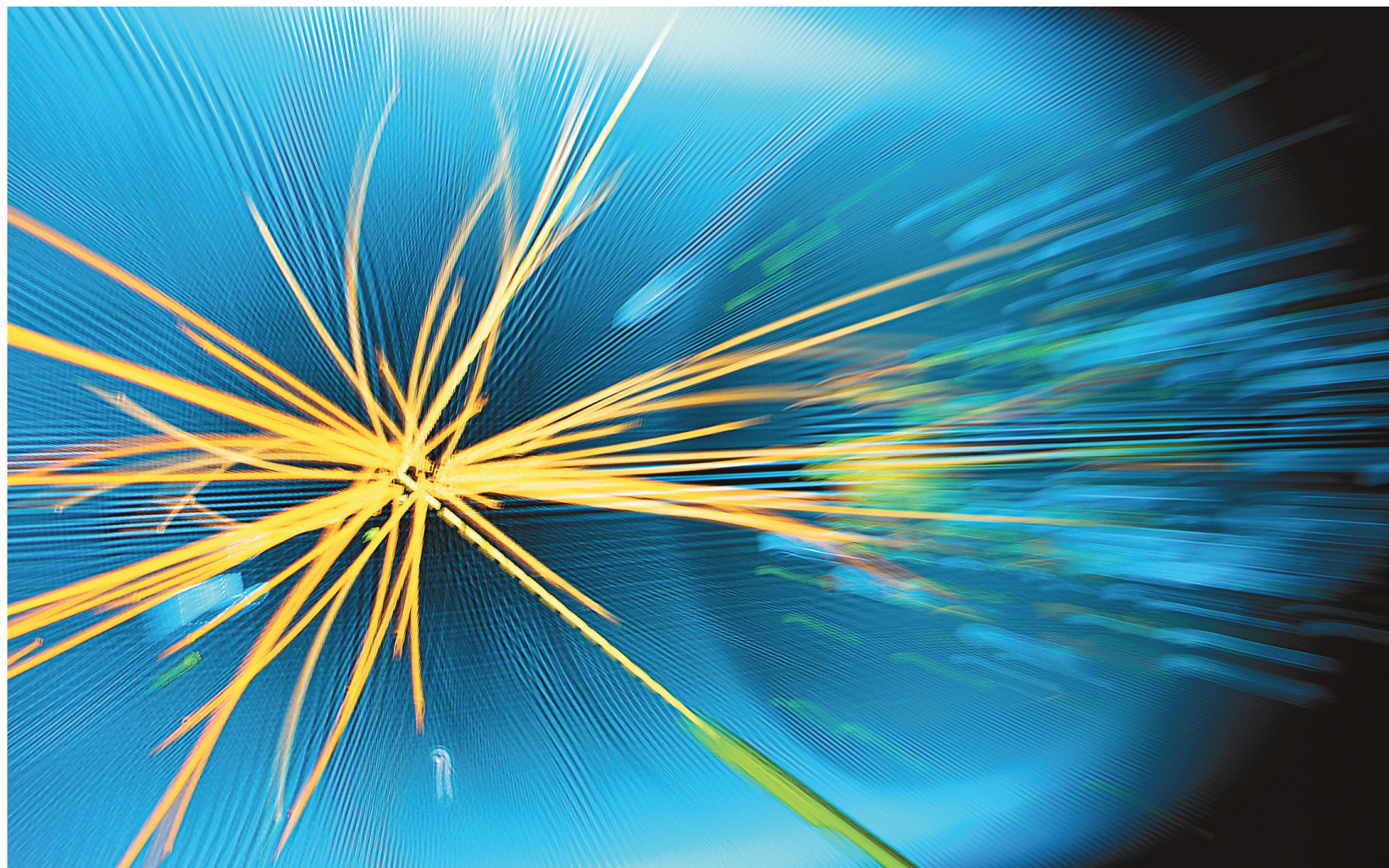
Une image montrant une collision de particules provoquée dans le Large Hadron Collider de l'Organisation européenne pour la recherche nucléaire.
